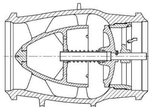
Рис. 2 Оссиметричный обратный клапан с присоединением под приварку (варианты см. рис. 1)
